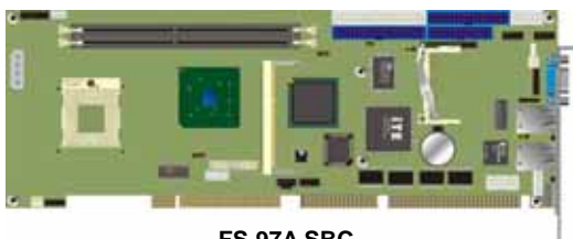
FS-97A SBC
